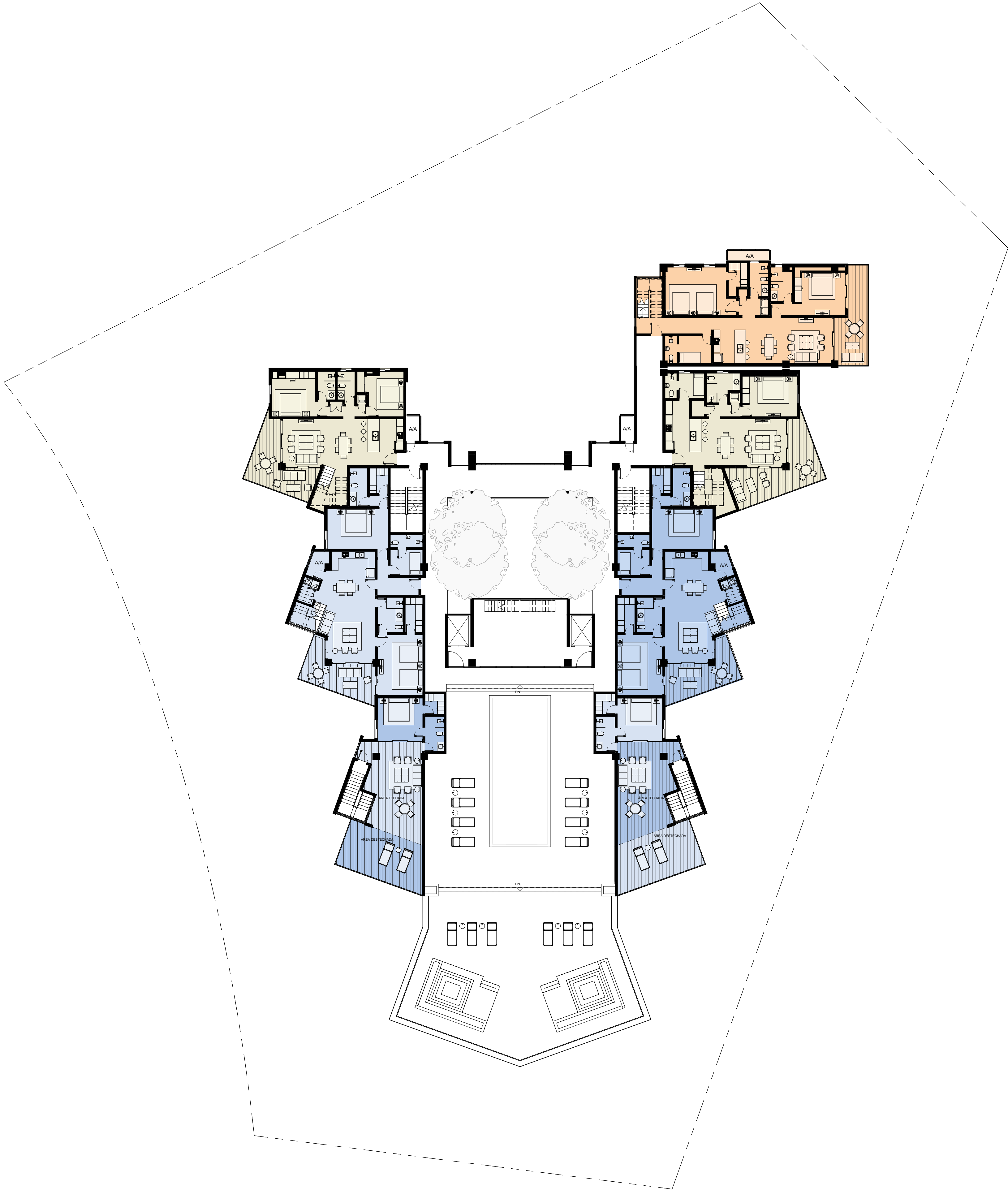
① NIVEL 5 1 : 200
