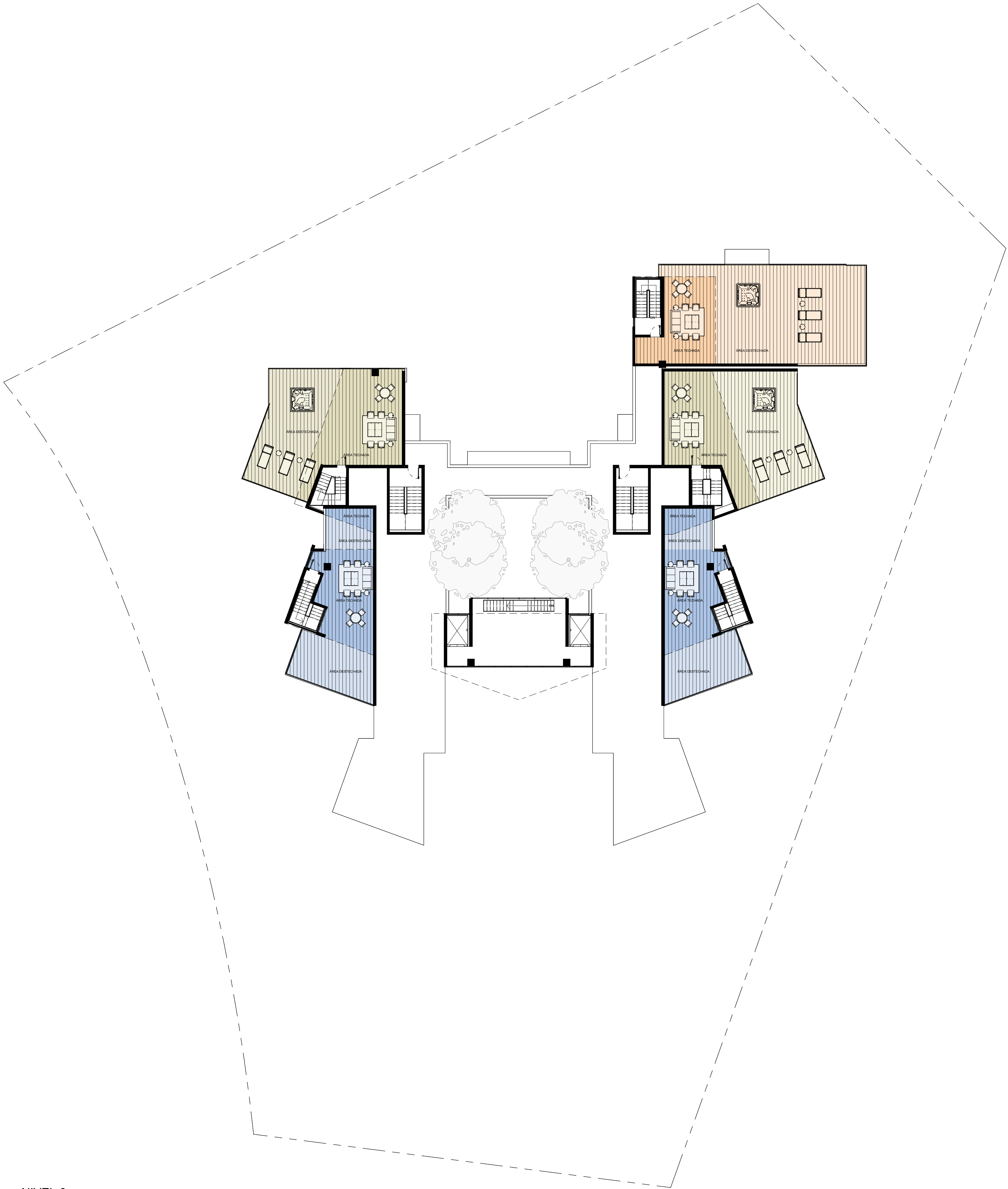
① NIVEL 6 1 : 200
